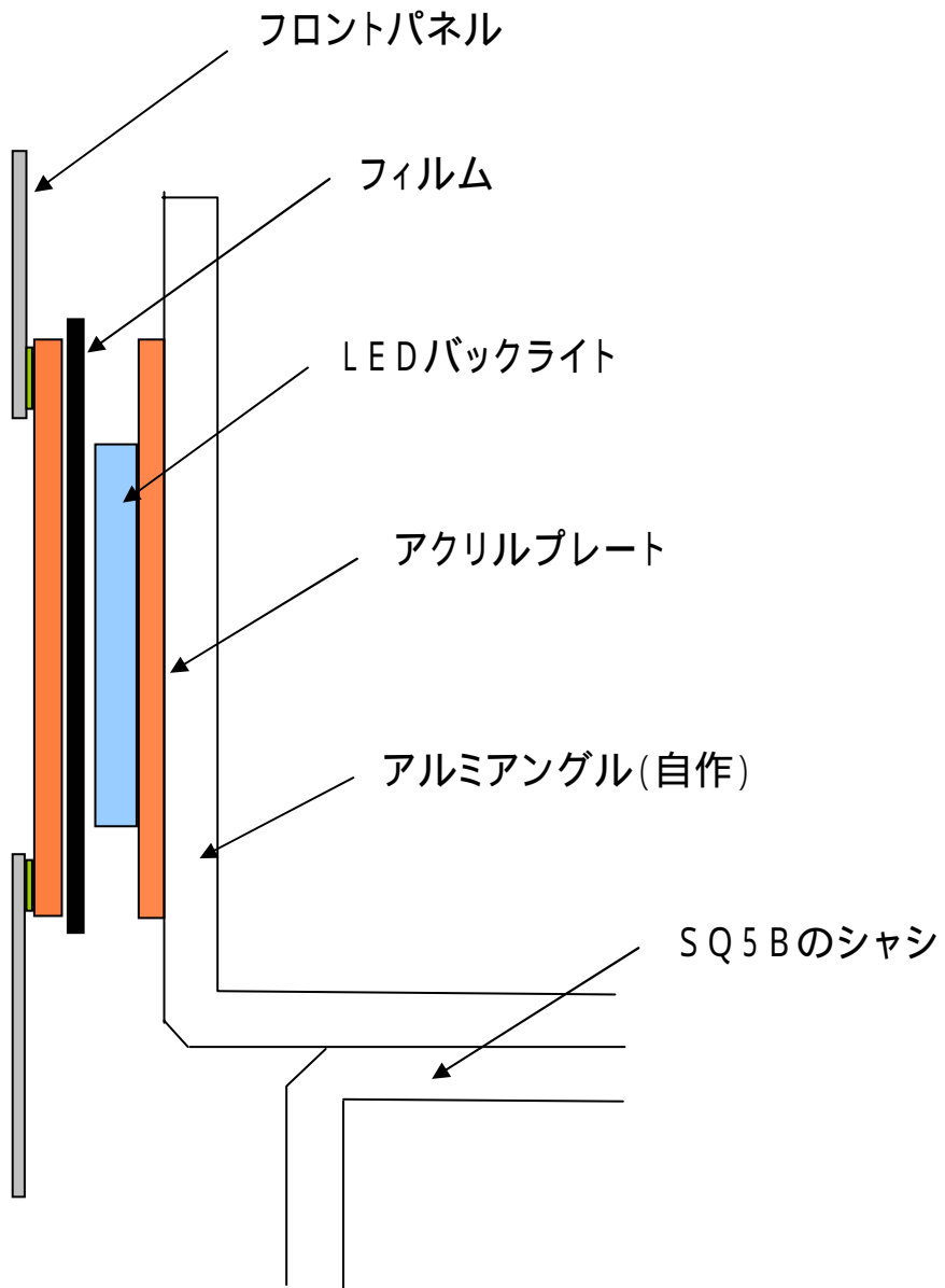
断面図
