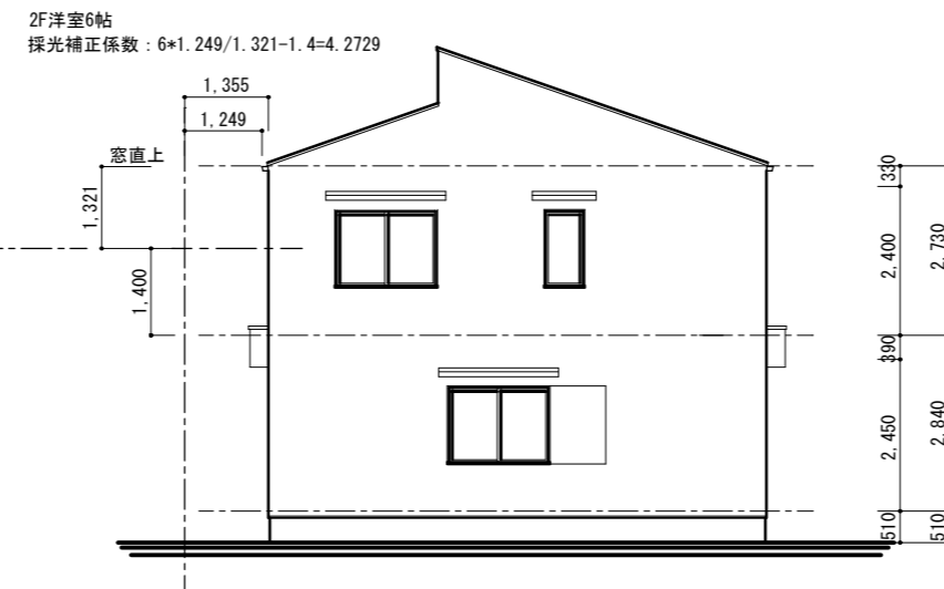
西側
