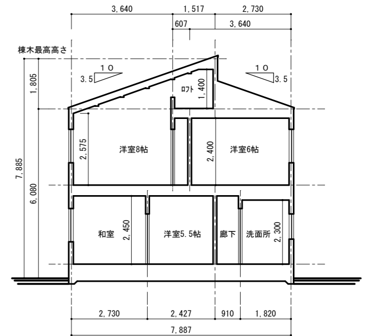
南北断面図
