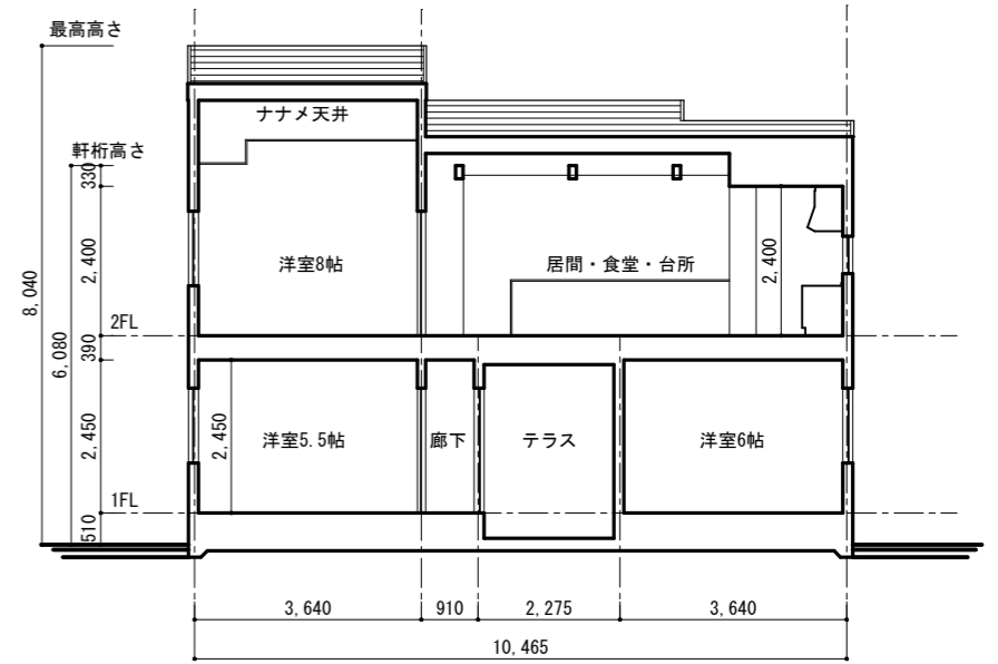
東西断面図
