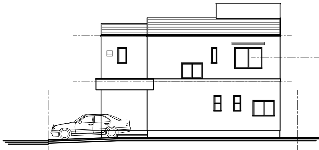
北側
