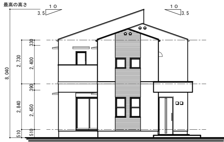
道路側
